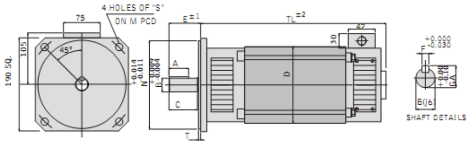
(V1-L, V2-L, V3-100B5)
