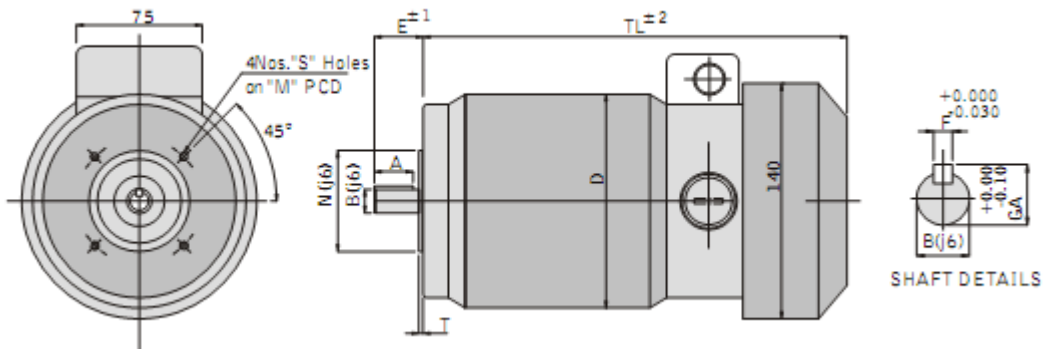
(M30-71B14, M3-71B14) IEC Flange
