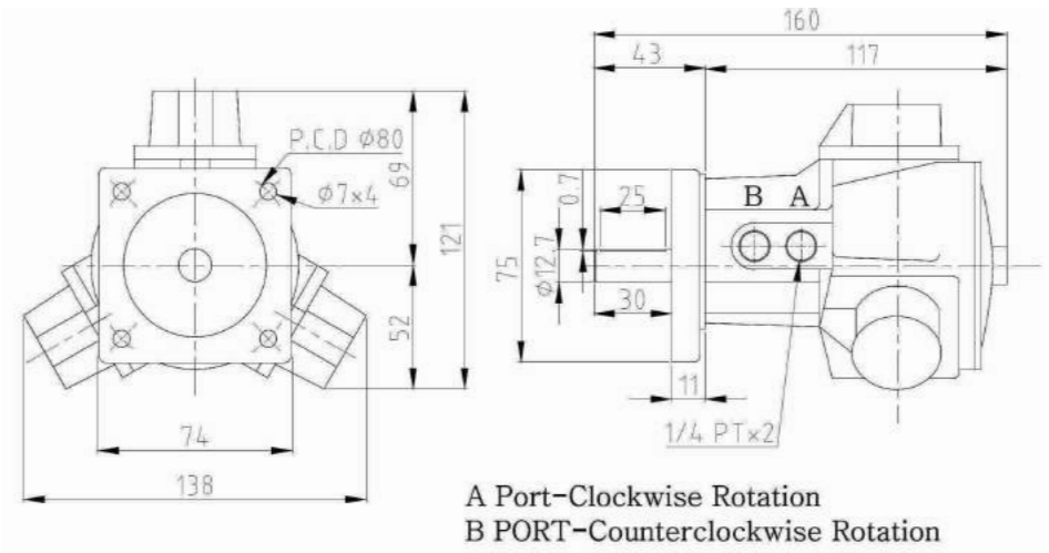
M2-F Face
