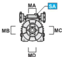
Posizione morsettiere e scatola di comando
