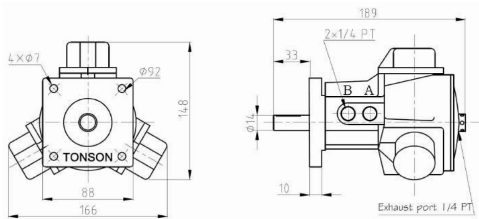
M4-F Face
