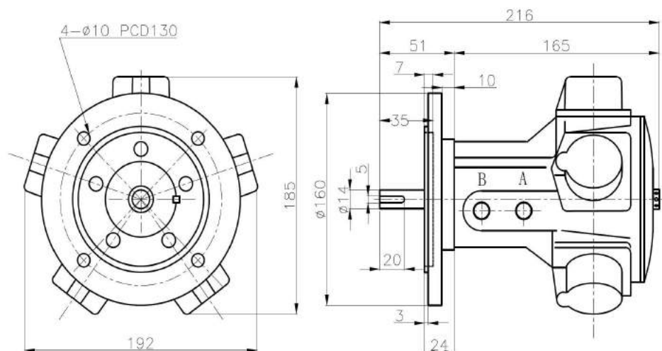
M6-I IEC D71
